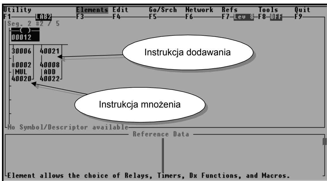
Rys. 10. Sieć 2 podprogramu
