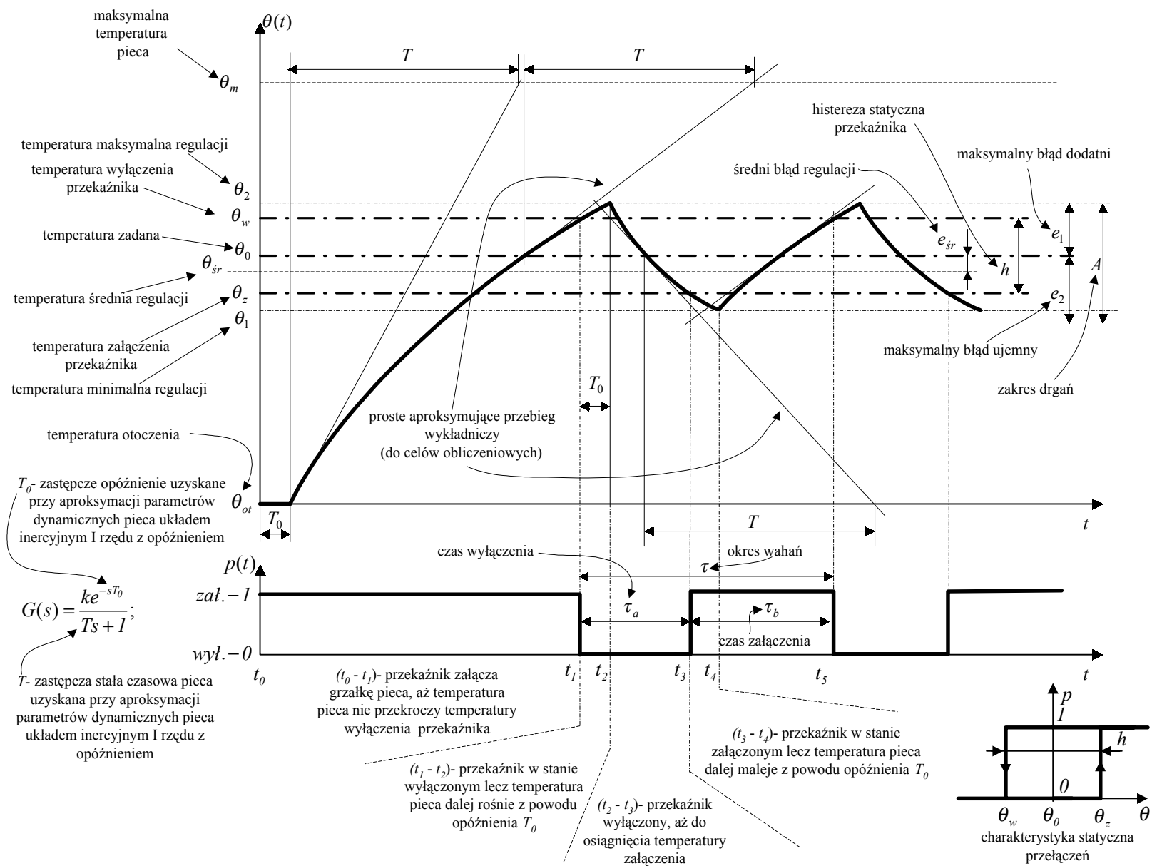
Rys. 6.5. Graficzna analiza pracy regulatora dwupołożeniowego regulującego temperaturę w piecu elektrycznym
